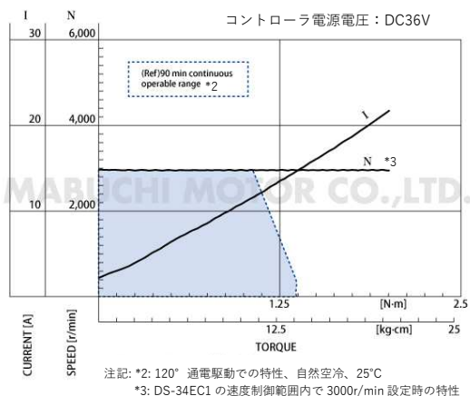
DS-34EC1 接続時 (180° 正弦波駆動)
